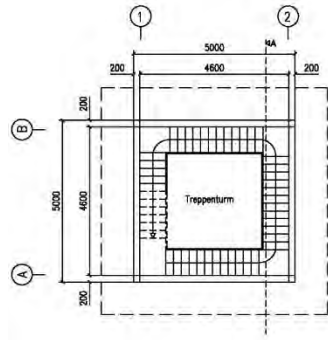
GRUNDRISS TREPPE
